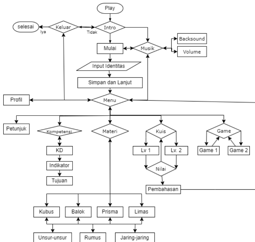
Gambar 2. Flowchart Media Pembelajaran BERUANG
